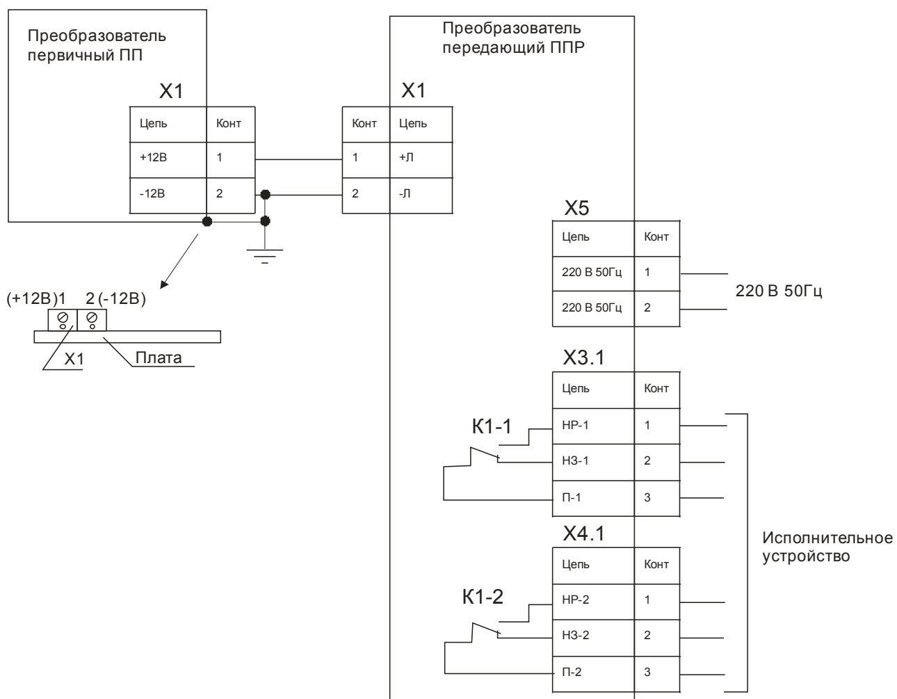
Рис. В.2 - Схема подключения ПРУ-5М (невзрывозащищенное исполнение)
