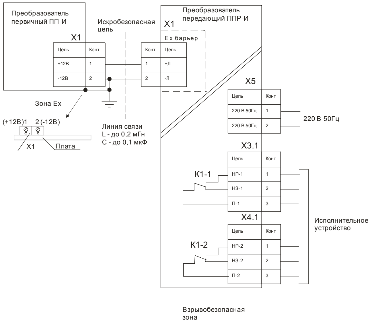
Рис. В.1 - Схема подключения ПРУ-5М-И (взрывозащищенное исполнение)
